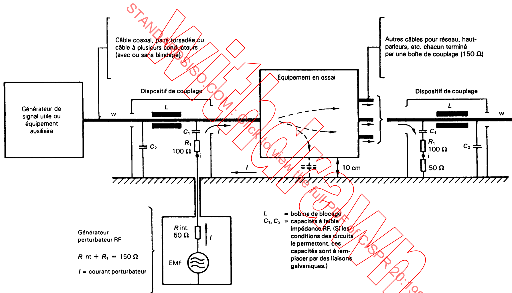
Figure 12 – Principe général de la méthode d'injection de courant (voir 5.4.2)
