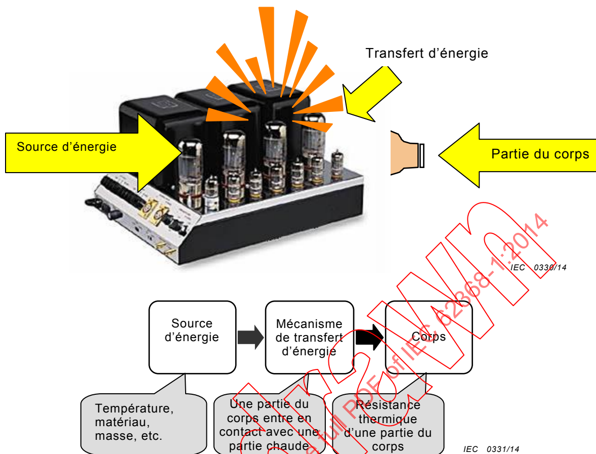
Figure 7 – Schéma et modèle pour les blessures dues à la chaleur
