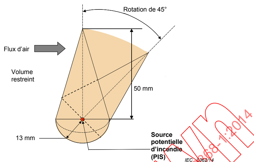
Figure 39 – Exigences de séparation en rotation causée par un flux d'air forcé
