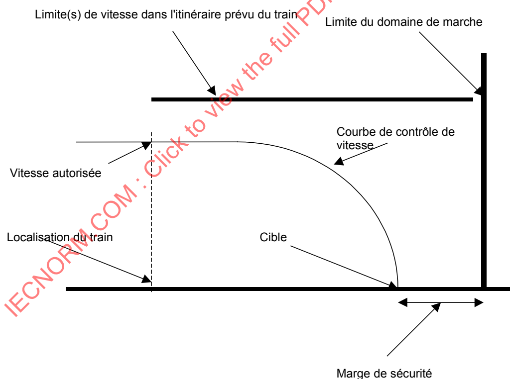
Figure 3 – Courbe de contrôle et supervision de la vitesse
