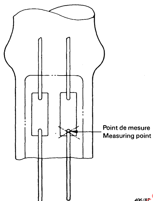
Fig. 8.- Point de fixation du thermocouple. Fixing point for thermocouple.
