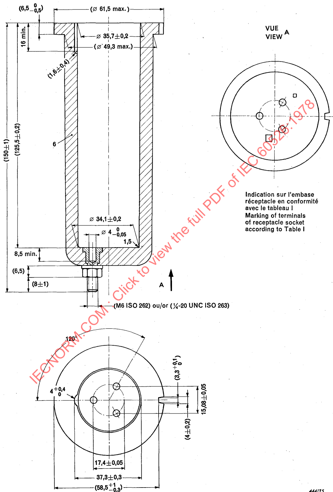
FIG. 2. — Embase réceptacle à trois conducteurs. Three-conductor receptacle socket.
