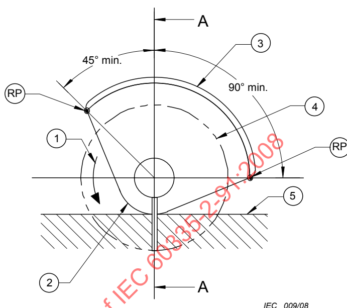
Figure 102b – Vue en direction de l'organe de coupe
