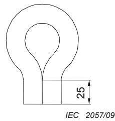
Figure 103 – Configuration du flexible pour le conditionnement à basse température
