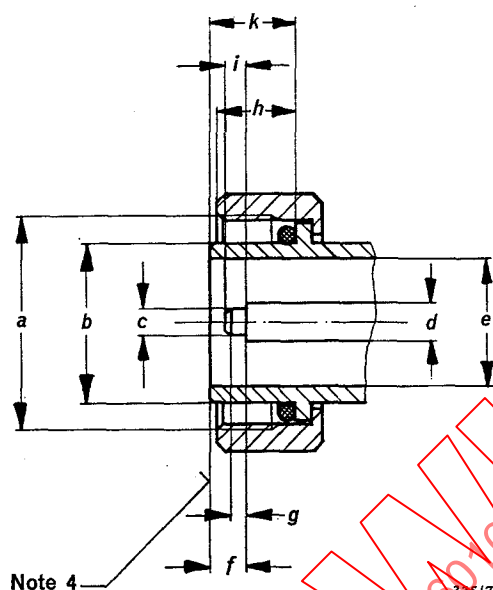
FIG. 1. — Connecteur avec contact central mâle (pour les dimensions, voir le tableau). Connector with pin centre contact (for dimensions, see table).
