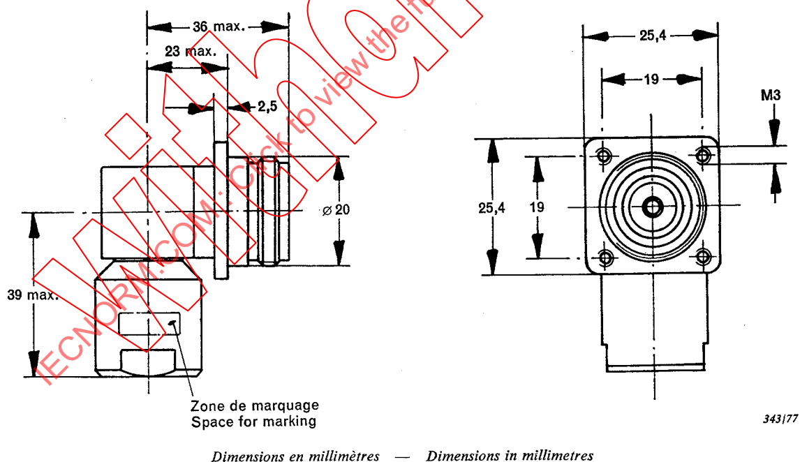
FIG. 9. — Prise à platine (coudée à angle droit, fixation au panneau par quatre trous avec sortie pour câble pour fréquences radioélectriques) avec contact femelle.
