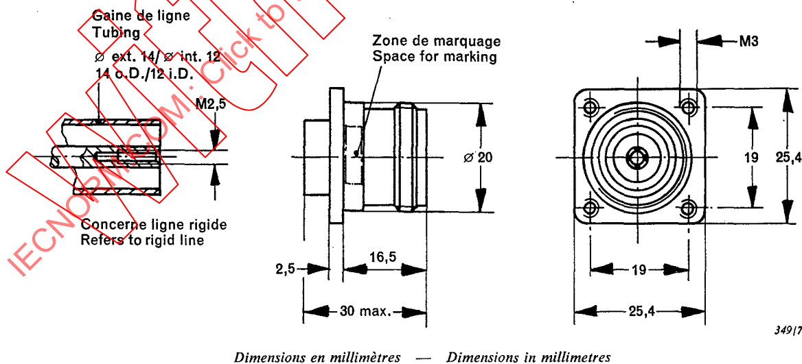
FIG. 15. — Prise à platine (fixation au panneau par quatre trous, pour lignes rigides) avec contact femelle. Fixed connector (4-hole panel mounting for rigid lines) with socket contact.
