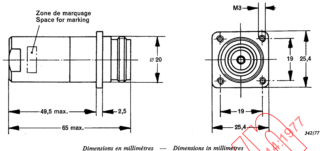
FIG. 8. — Prise à platine (droite, fixation au panneau par quatre trous avec sortie pour câbles pour fréquences radioélectriques) avec contact femelle.
