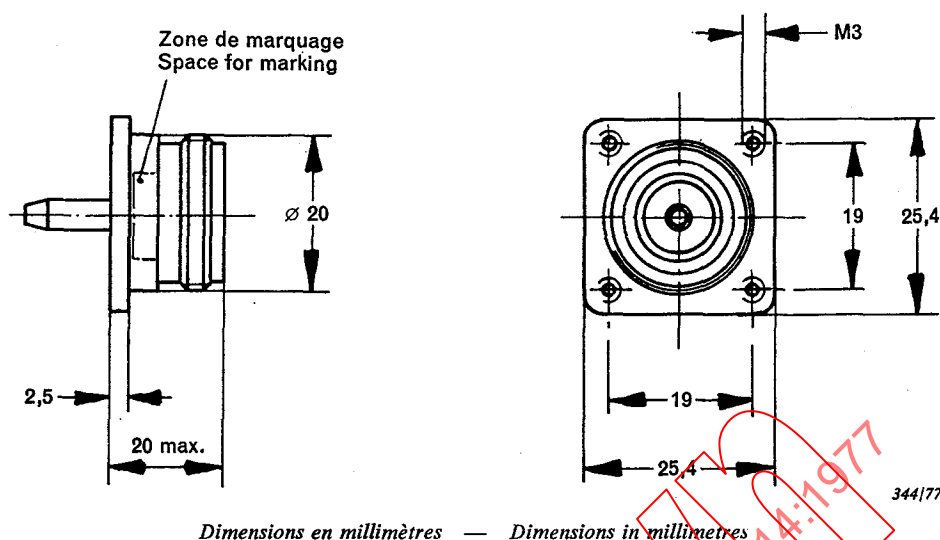
FIG. 10. — Embase à platine (fixation au panneau par quatre trous, avec cosse à souder) avec contact femelle.
