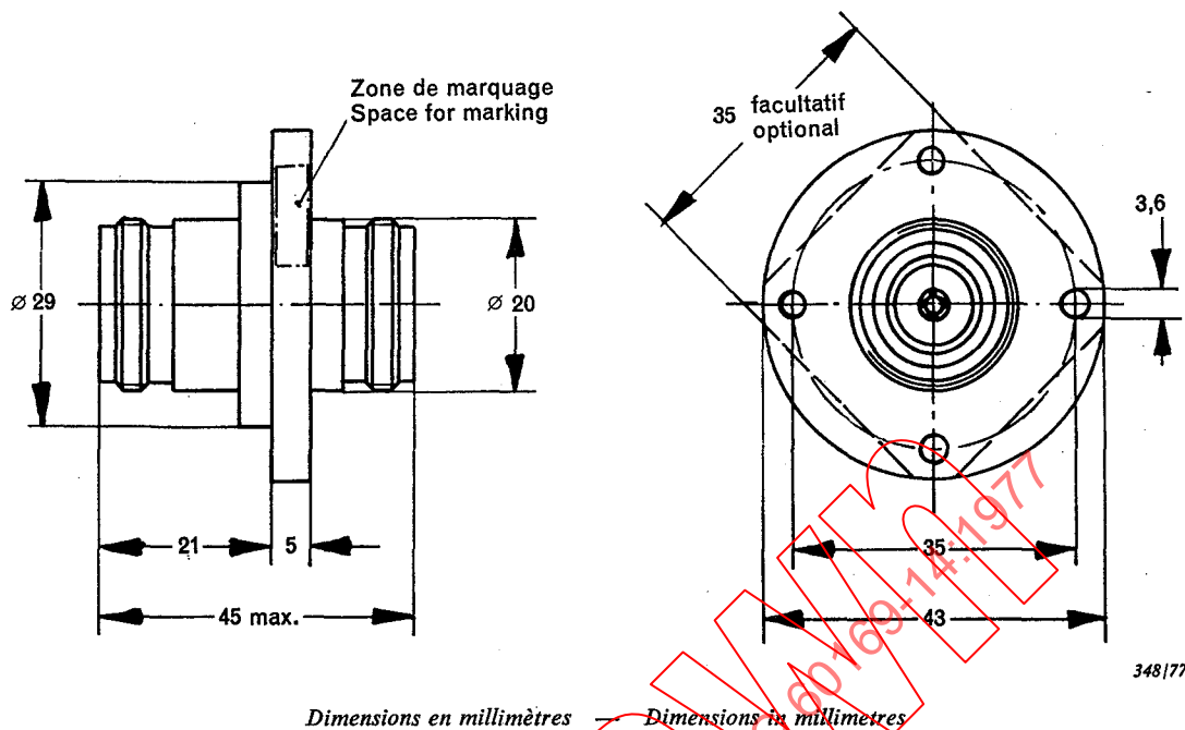
FIG. 14. — Raccord fixe (fixation au panneau par quatre trous) avec contacts femelle-femelle. Fixed adaptor (4-hole panel mounting) with socket-socket contacts.
